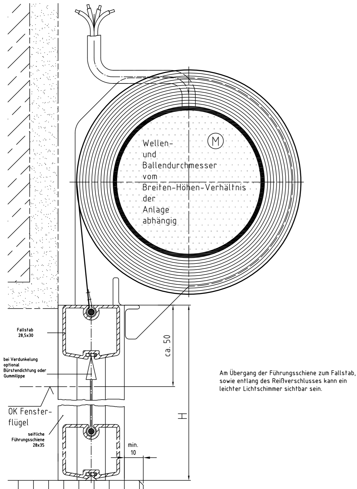
Zeichnung ZIP-MO – Querschnitt Systemskizze | ohne Maßstab | sämtliche Angaben in mm
