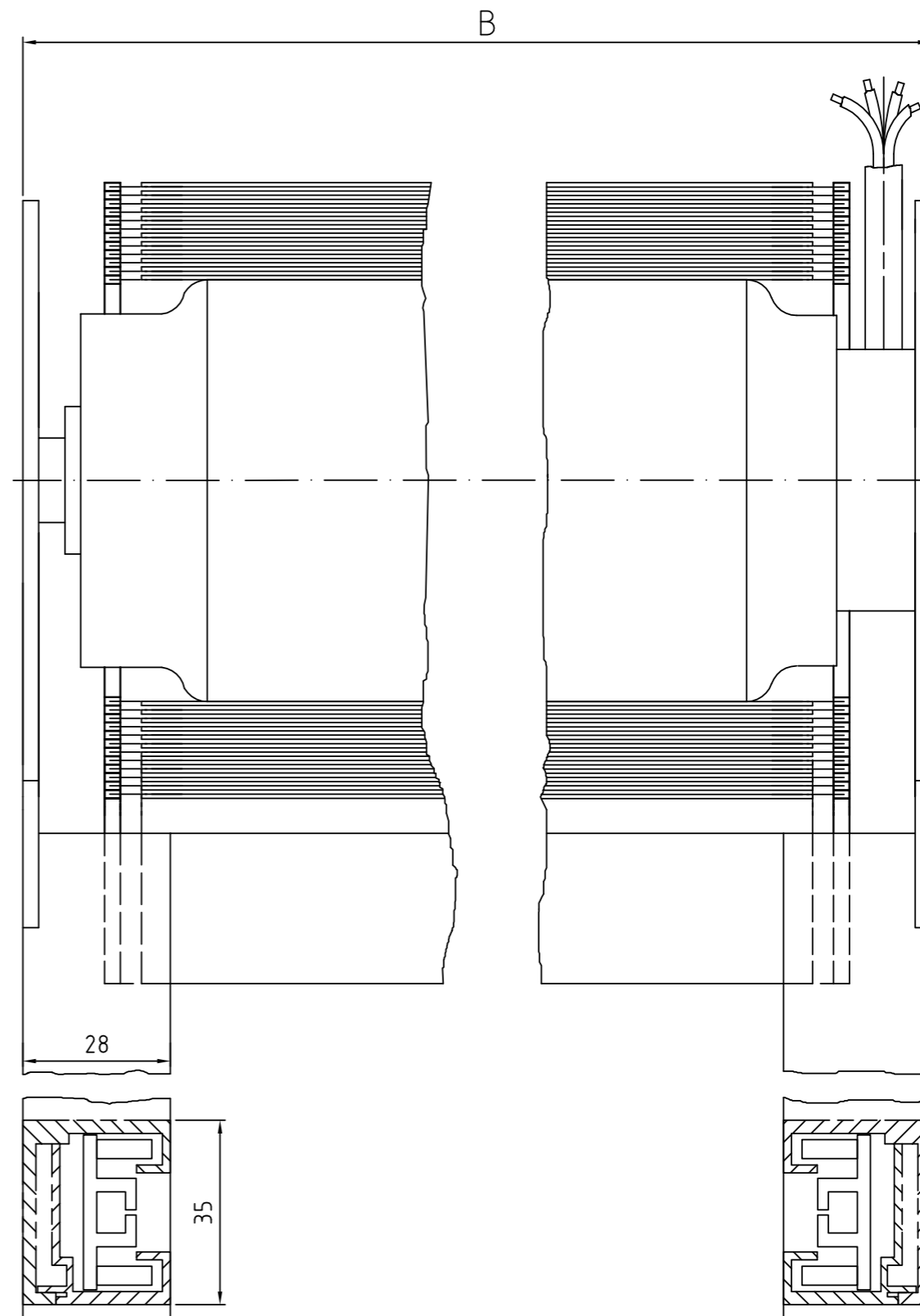
Zeichnung ZIP-MO – Längsschnitt Systemskizze | ohne Maßstab | sämtliche Angaben in mm
