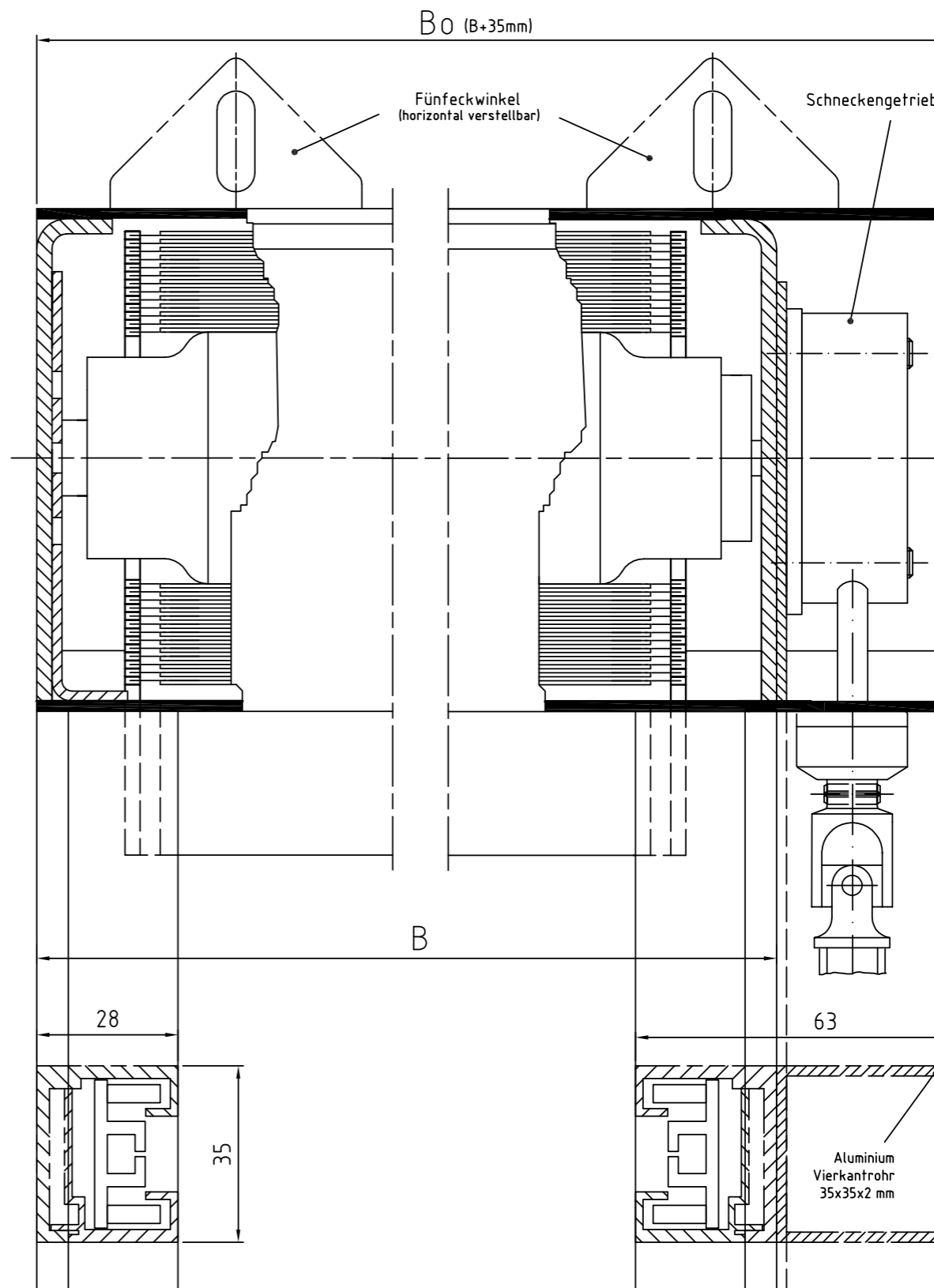
Zeichnung ZIP-GQ 100 – Längsschnitt Systemskizze | ohne Maßstab | sämtliche Angaben in mm
