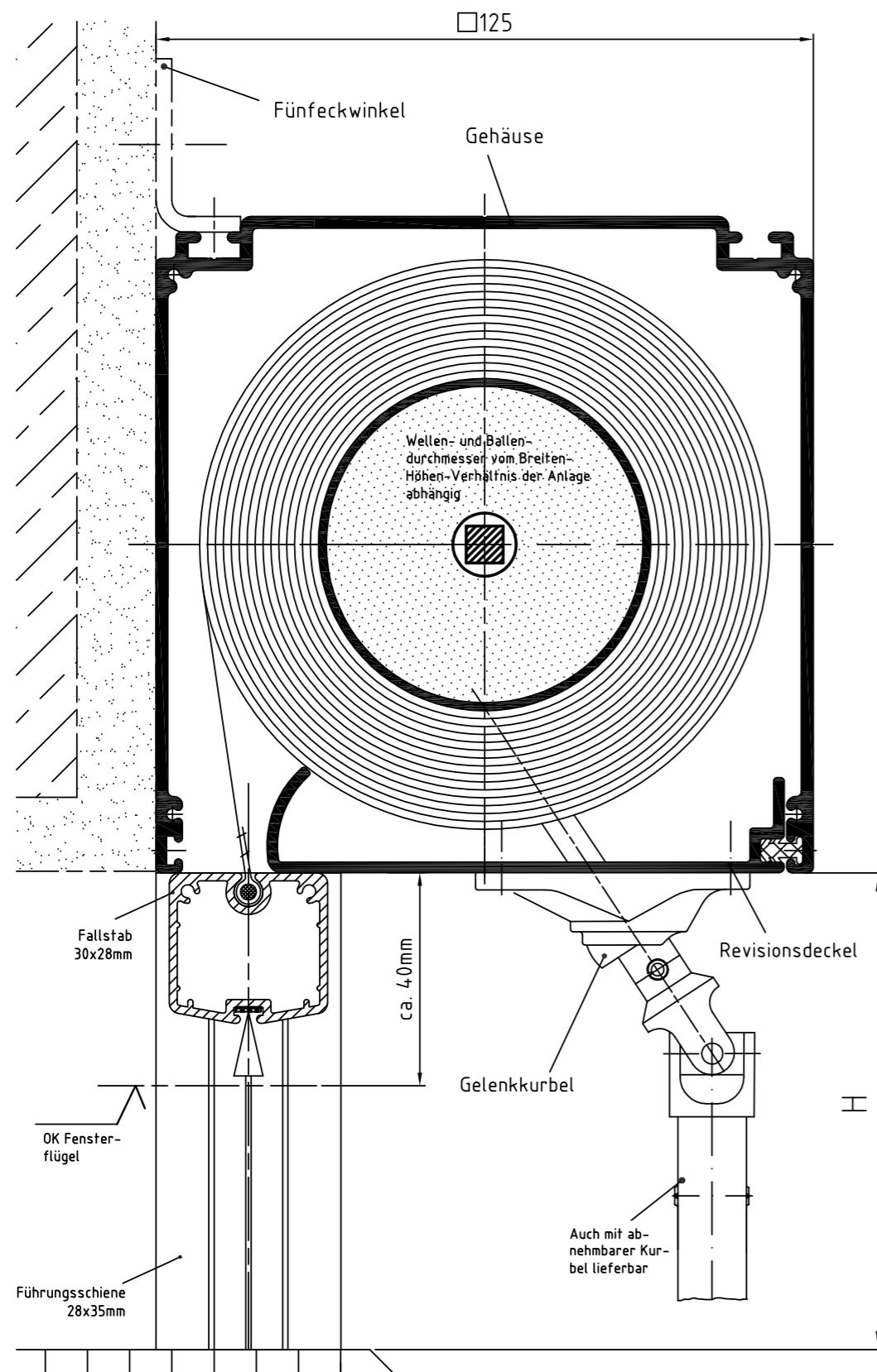
Zeichnung ZIP-GQ 125 – Querschnitt Systemskizze | ohne Maßstab | sämtliche Angaben in mm
