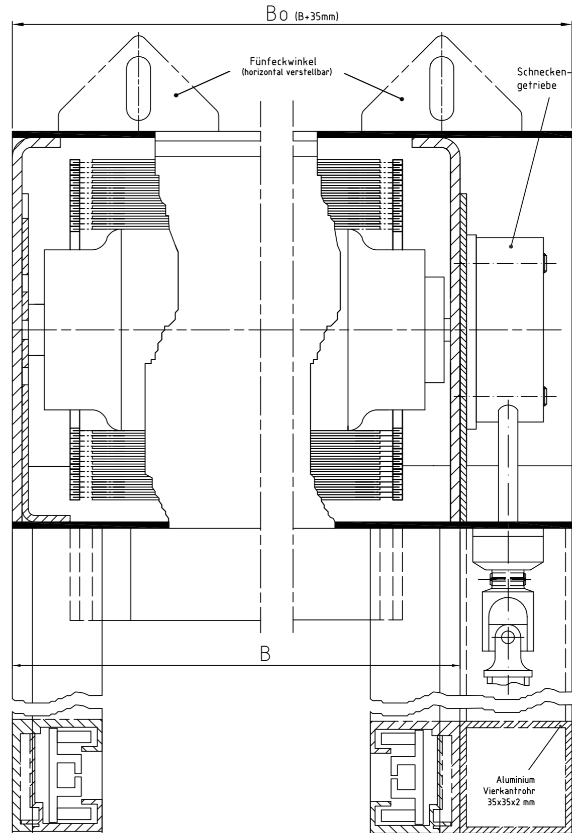
Zeichnung ZIP-GQ 125 – Längsschnitt Systemskizze | ohne Maßstab | sämtliche Angaben in mm
