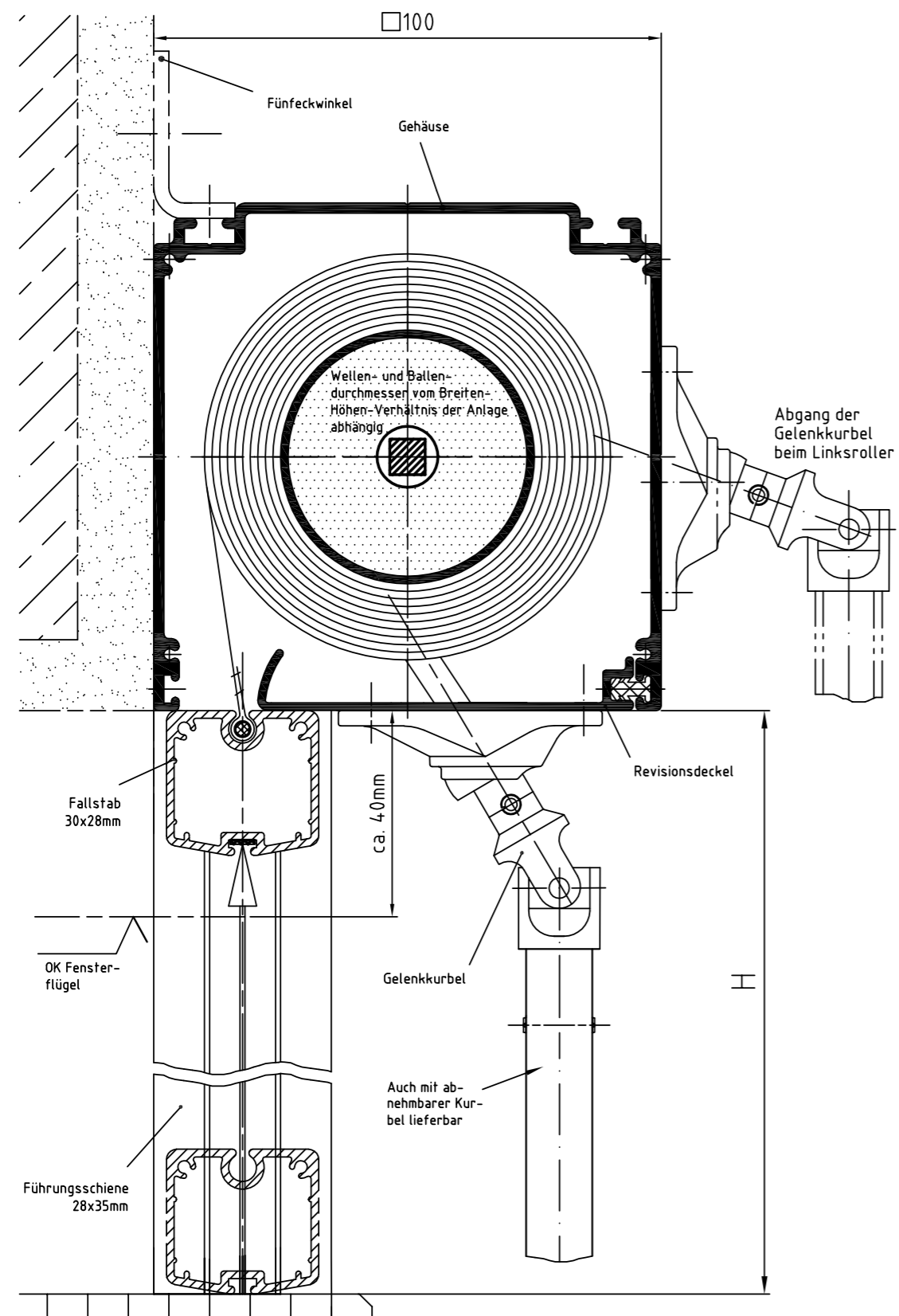
Zeichnung ZIP-GQ 100 – Querschnitt Systemskizze | ohne Maßstab | sämtliche Angaben in mm
