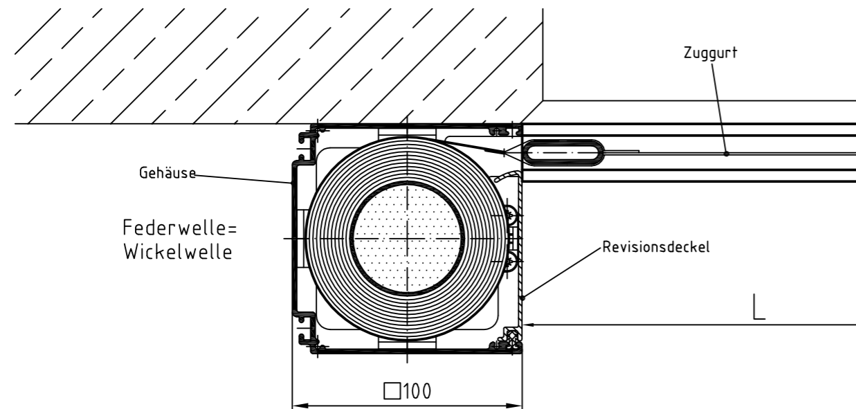
Zeichnung W-U-GZ-MQ 100 – Querschnitt Systemskizze | ohne Maßstab | sämtliche Angaben in mm
