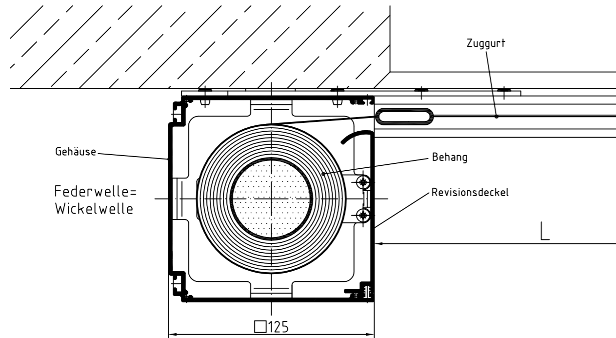
Zeichnung W-U-GZ-MQ 125 – Querschnitt Systemskizze | ohne Maßstab | sämtliche Angaben in mm
