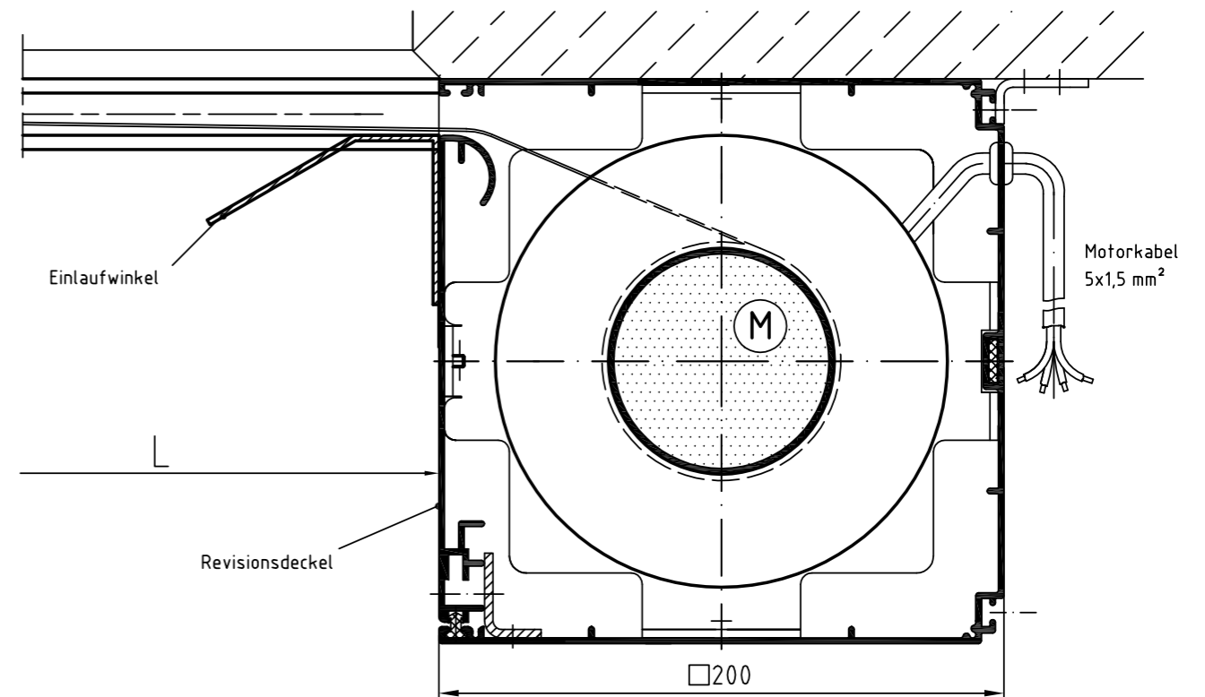
Zeichnung W-U-GZ-MQ 200 – Längsschnitt Systemskizze | ohne Maßstab | sämtliche Angaben in mm
