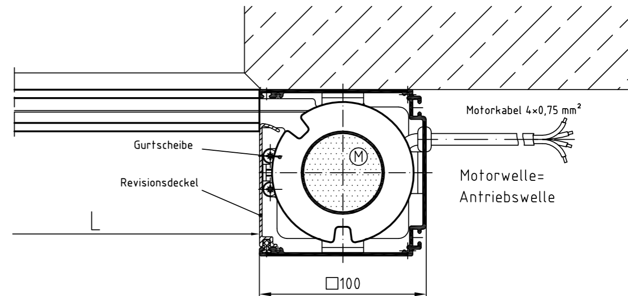
Zeichnung W-U-GZ-MQ 100 – Längsschnitt Systemskizze | ohne Maßstab | sämtliche Angaben in mm
