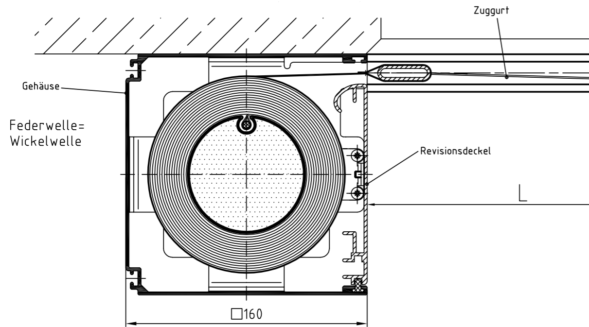
Zeichnung W-U-GZ-MQ 160 – Querschnitt Systemskizze | ohne Maßstab | sämtliche Angaben in mm
