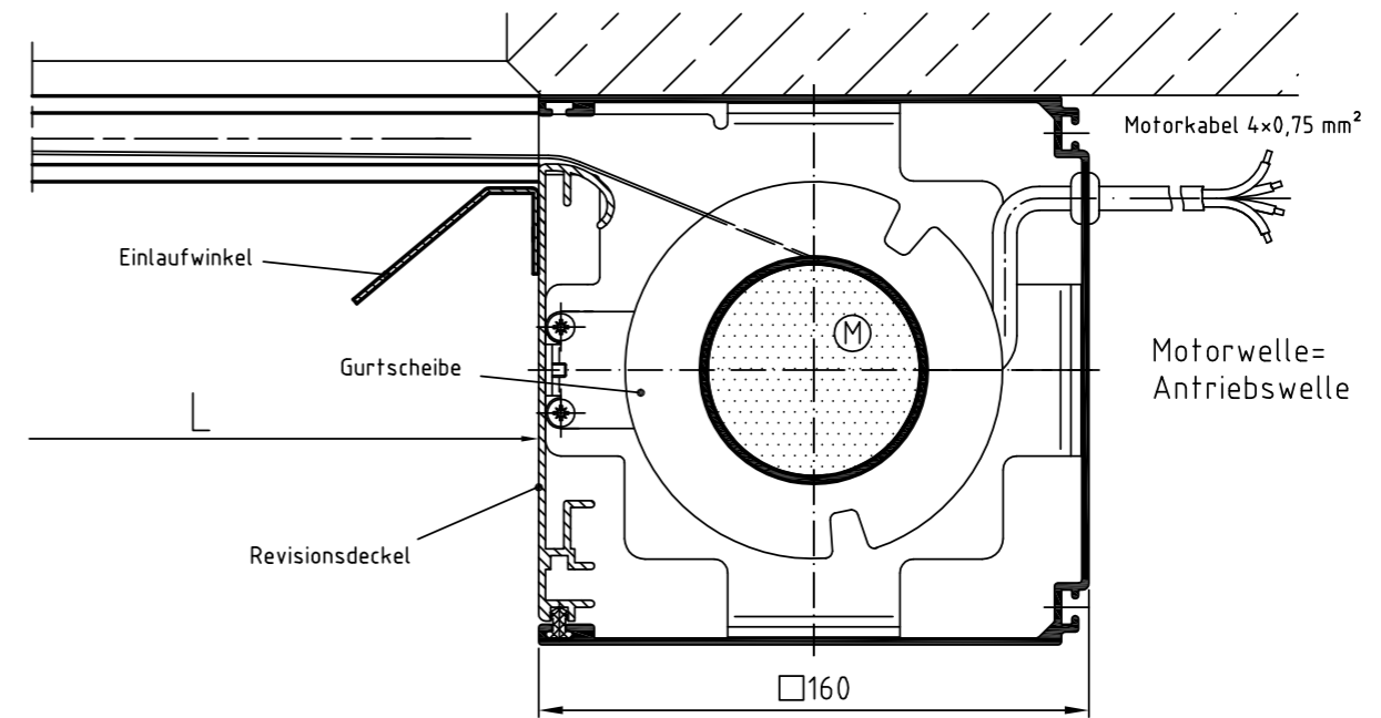
Zeichnung W-U-GZ-MQ 160 – Längsschnitt Systemskizze | ohne Maßstab | sämtliche Angaben in mm
