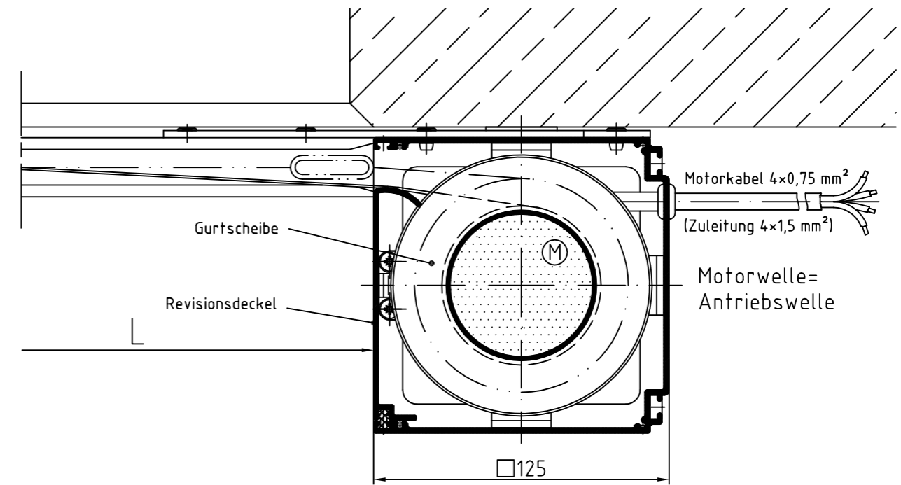
Zeichnung W-U-GZ-MQ 125 – Längsschnitt Systemskizze | ohne Maßstab | sämtliche Angaben in mm
