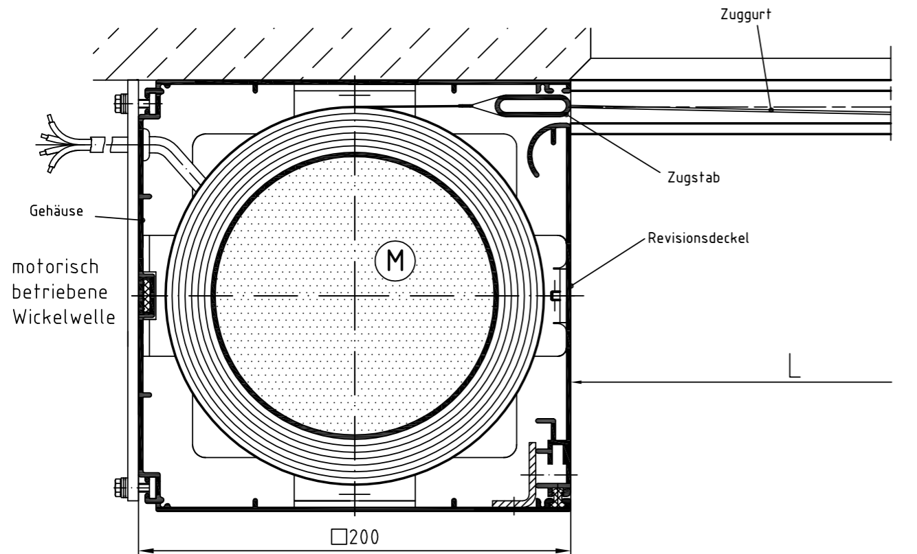
Zeichnung W-U-GZ-MQ 200 – Querschnitt Systemskizze | ohne Maßstab | sämtliche Angaben in mm
