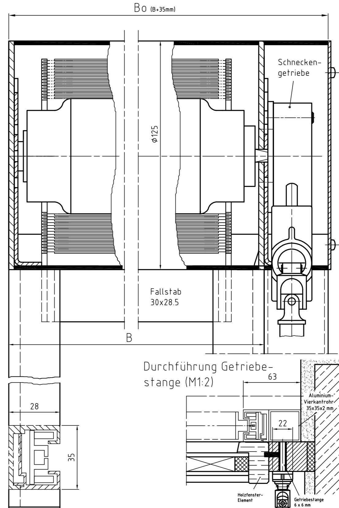
Zeichnung SM-ZIP-GR – Längsschnitt Systemskizze | ohne Maßstab | sämtliche Angaben in mm
