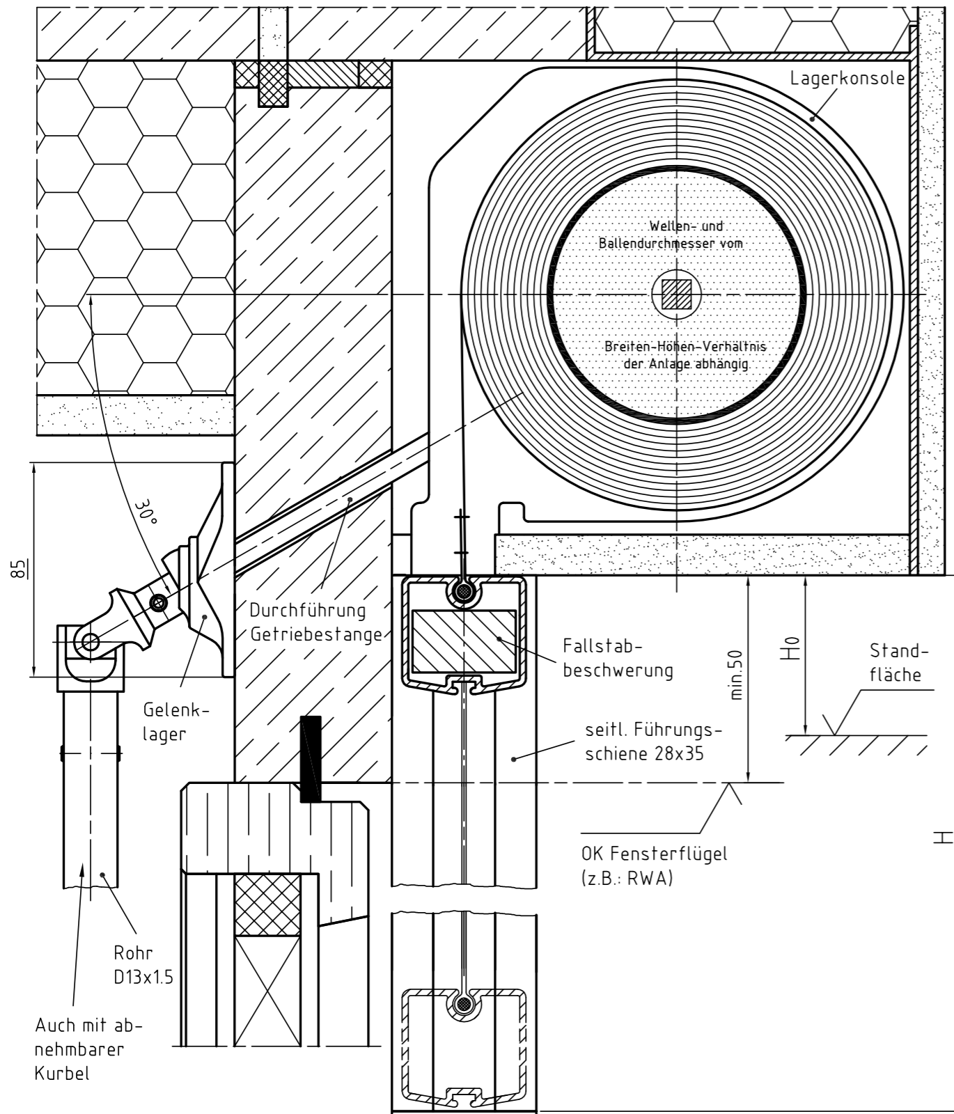
Zeichnung SM-ZIP-GO – Querschnitt Systemskizze | ohne Maßstab | sämtliche Angaben in mm
