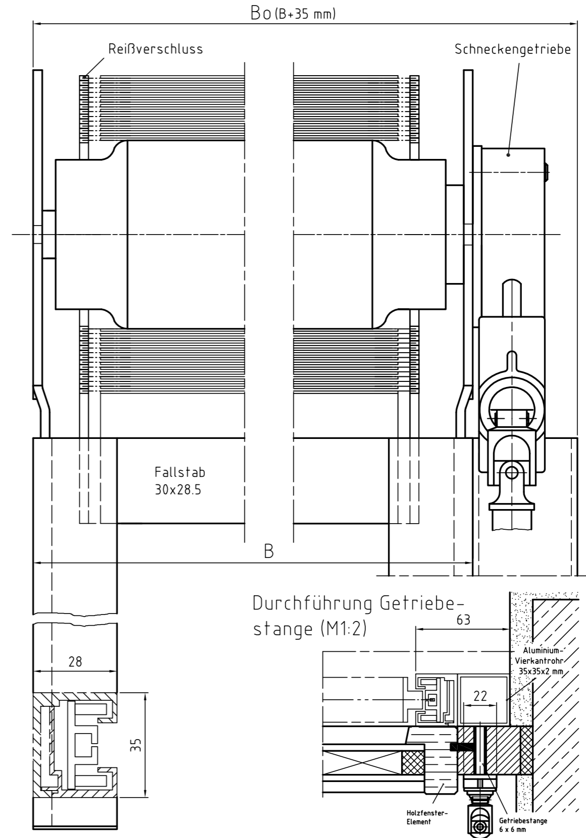
Zeichnung SM-ZIP-GO – Längsschnitt Systemskizze | ohne Maßstab | sämtliche Angaben in mm
