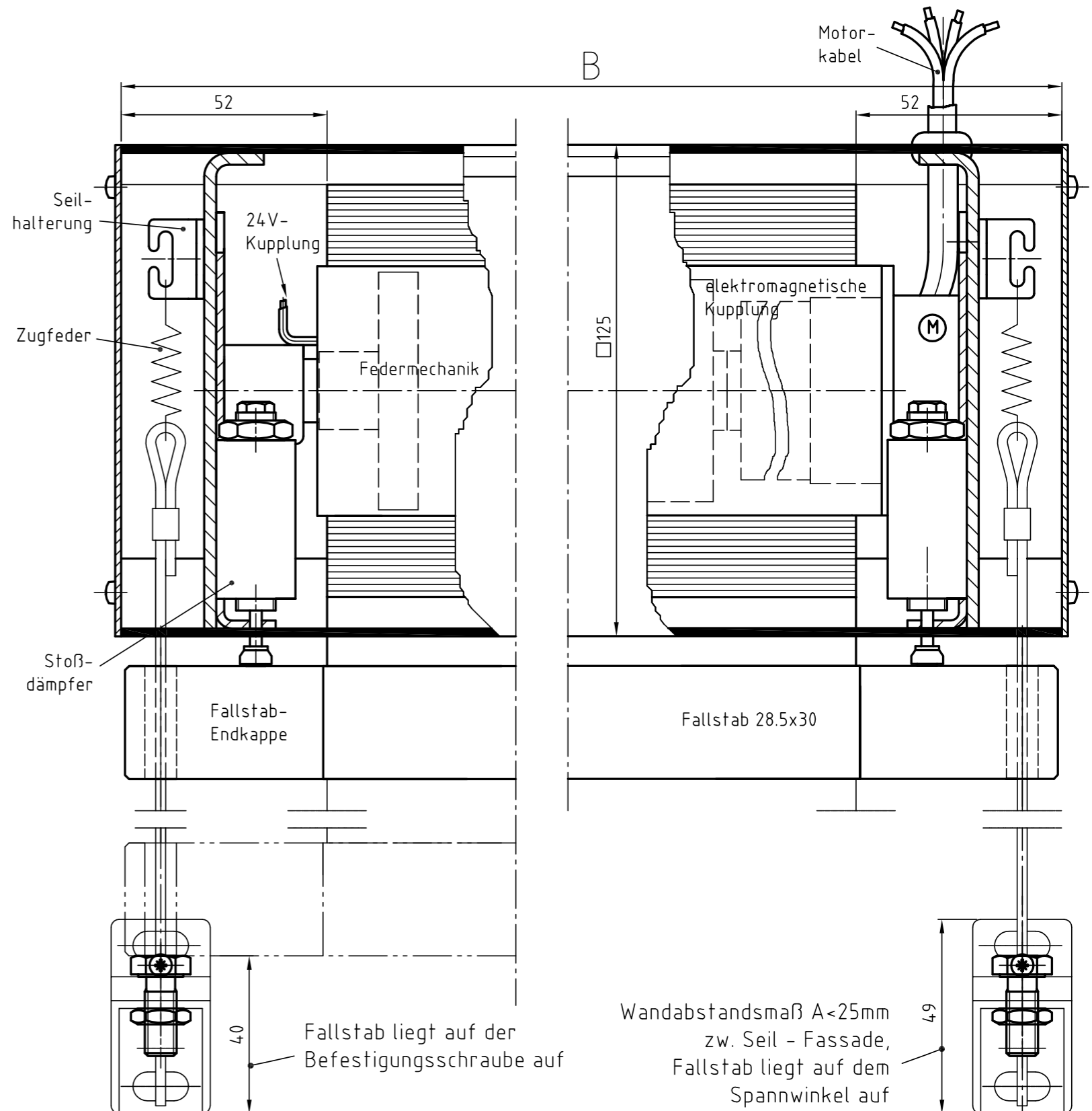
Zeichnung R2-K-MQ 125 – Längsschnitt Systemskizze | ohne Maßstab | sämtliche Angaben in mm
