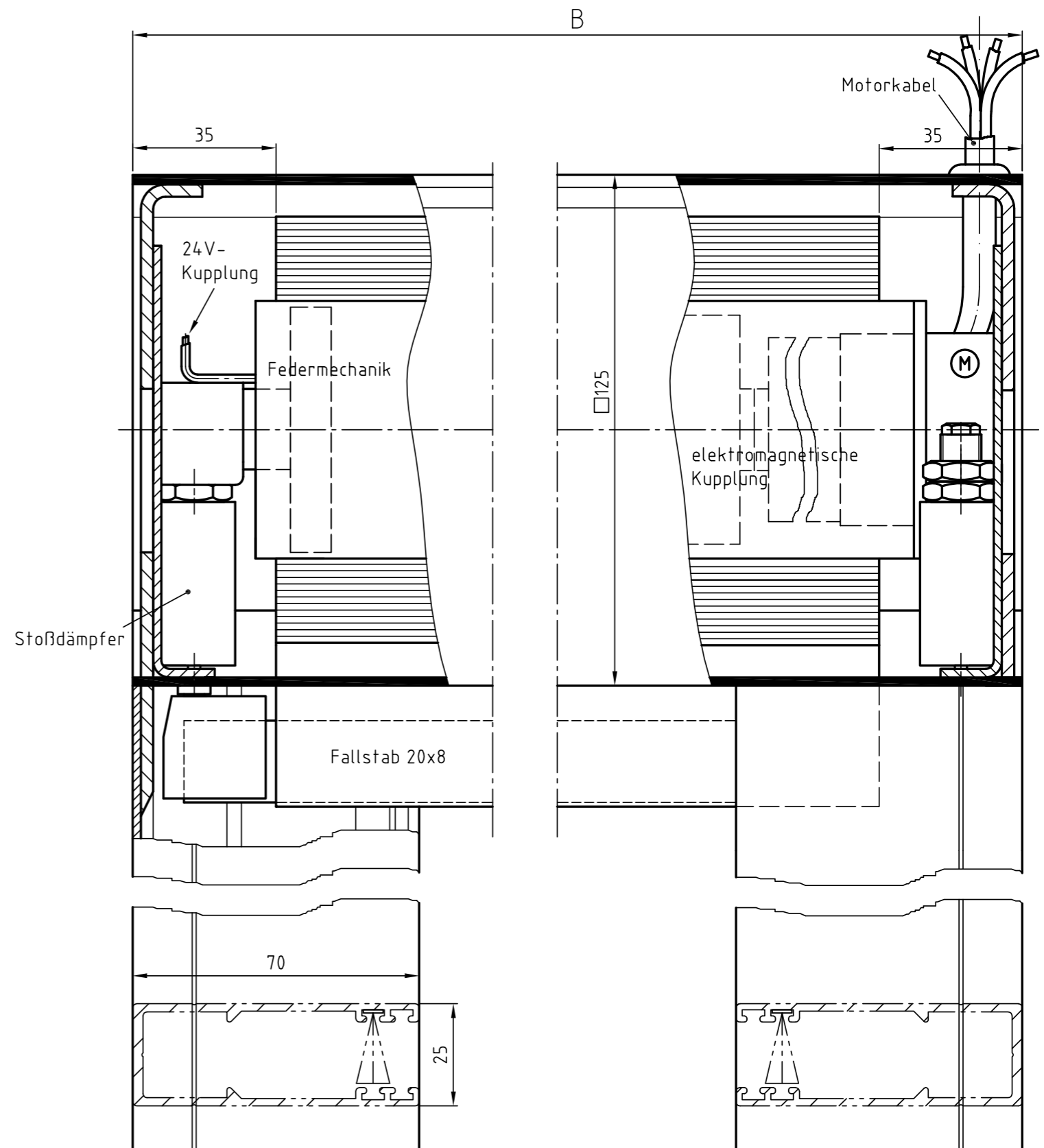
Zeichnung R2-K-MQ 125 – Längsschnitt Systemskizze | ohne Maßstab | sämtliche Angaben in mm
