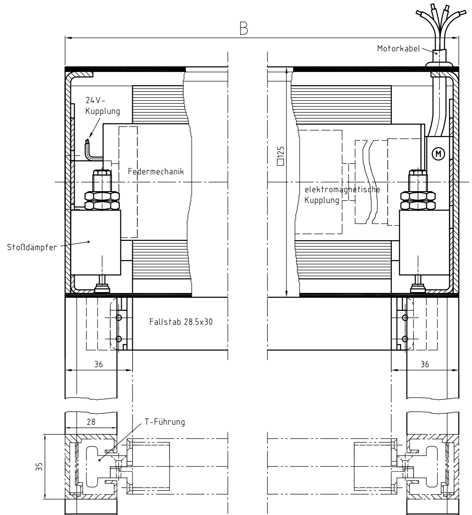
Zeichnung R1-K-MQ 125 – Längsschnitt Systemskizze | ohne Maßstab | sämtliche Angaben in mm
