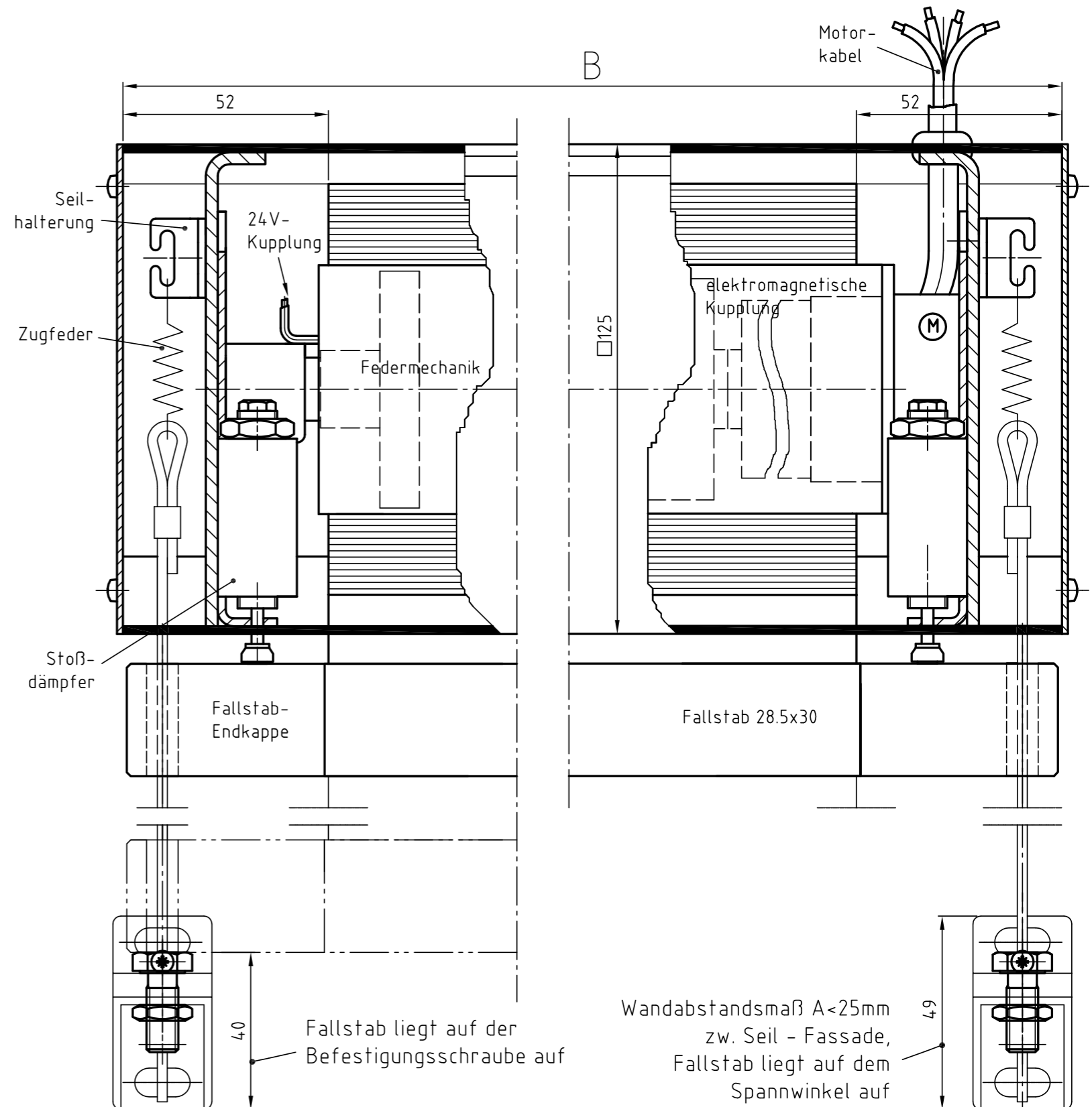
Zeichnung R1-K-MQ 125 – Längsschnitt Systemskizze | ohne Maßstab | sämtliche Angaben in mm
