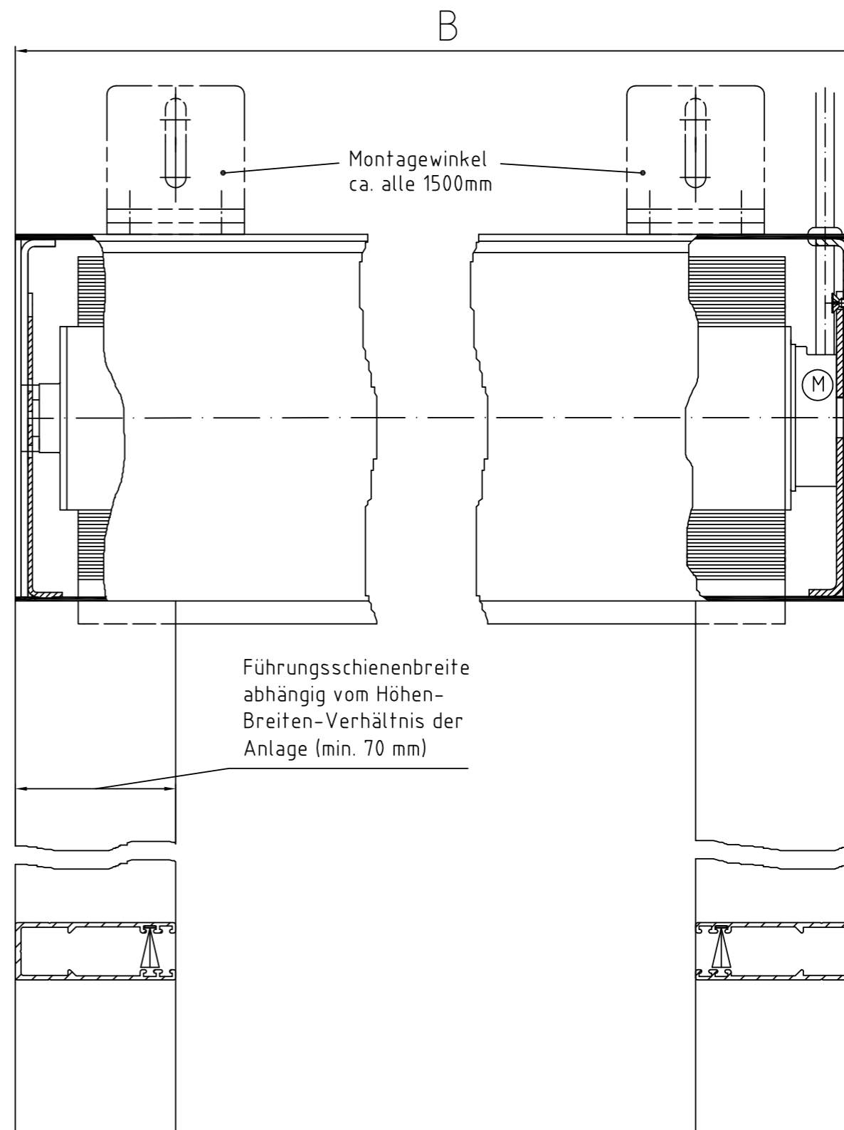
Zeichnung MQ 160 – Längsschnitt Systemskizze | ohne Maßstab | sämtliche Angaben in mm
