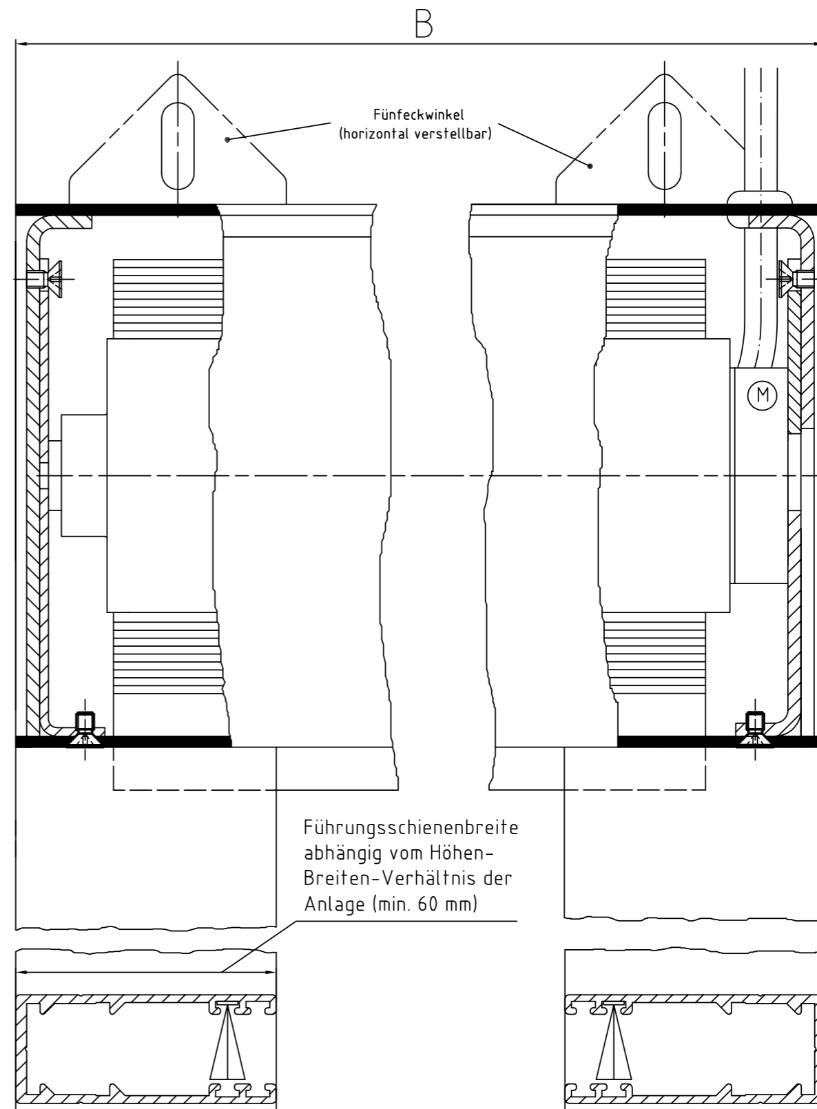
Zeichnung MQ 125 – Längsschnitt Systemskizze | ohne Maßstab | sämtliche Angaben in mm
