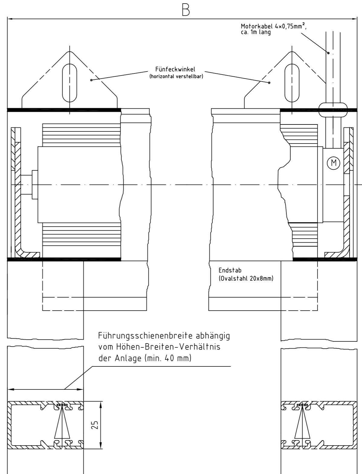
Zeichnung MQ 80 – Längsschnitt Systemskizze | ohne Maßstab | sämtliche Angaben in mm
