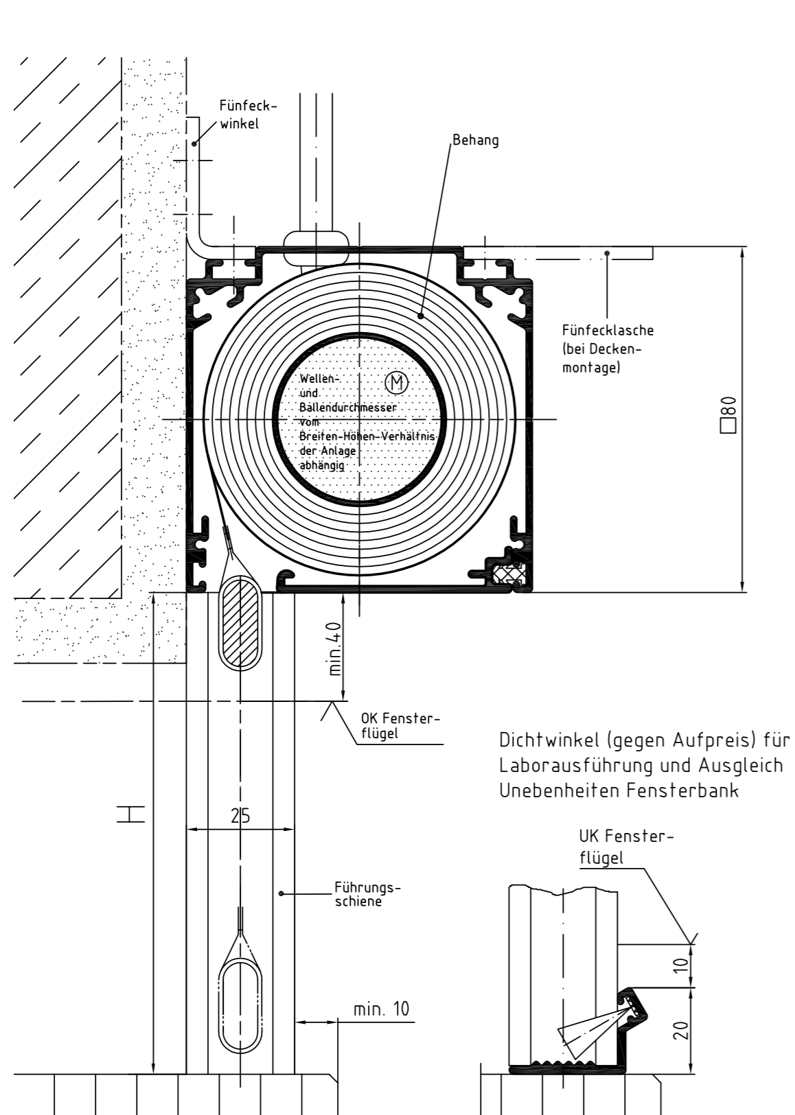
Zeichnung MQ 80 – Querschnitt Systemskizze | ohne Maßstab | sämtliche Angaben in mm
