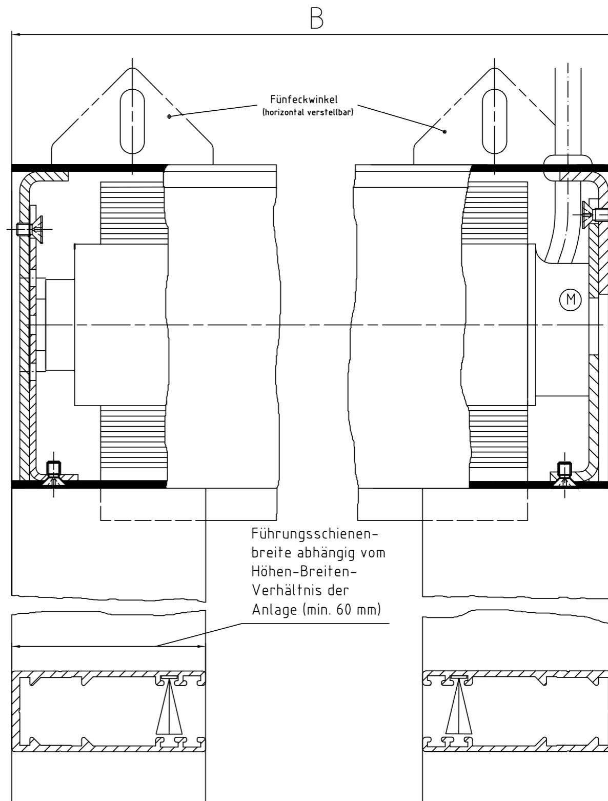
Zeichnung MQ 100 – Längsschnitt Systemskizze | ohne Maßstab | sämtliche Angaben in mm
