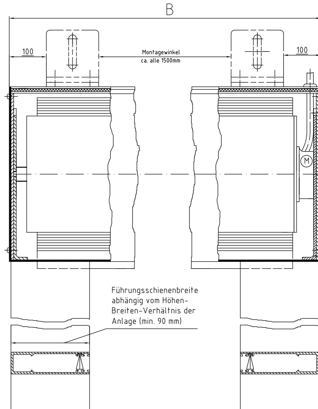
Zeichnung MQ 200 – Längsschnitt Systemskizze | ohne Maßstab | sämtliche Angaben in mm
