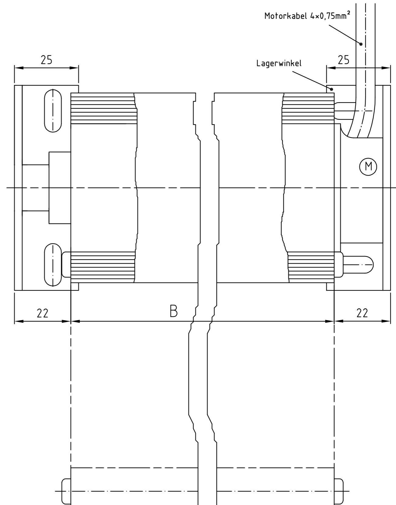
Zeichnung L-MO – Längsschnitt Systemskizze | ohne Maßstab | sämtliche Angaben in mm
