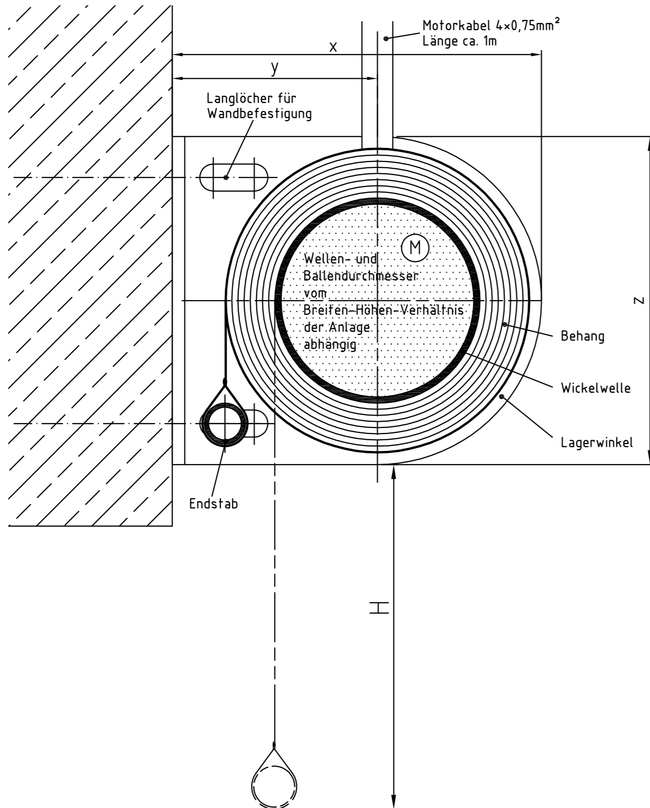
Zeichnung L-MO – Querschnitt Systemskizze | ohne Maßstab | sämtliche Angaben in mm
