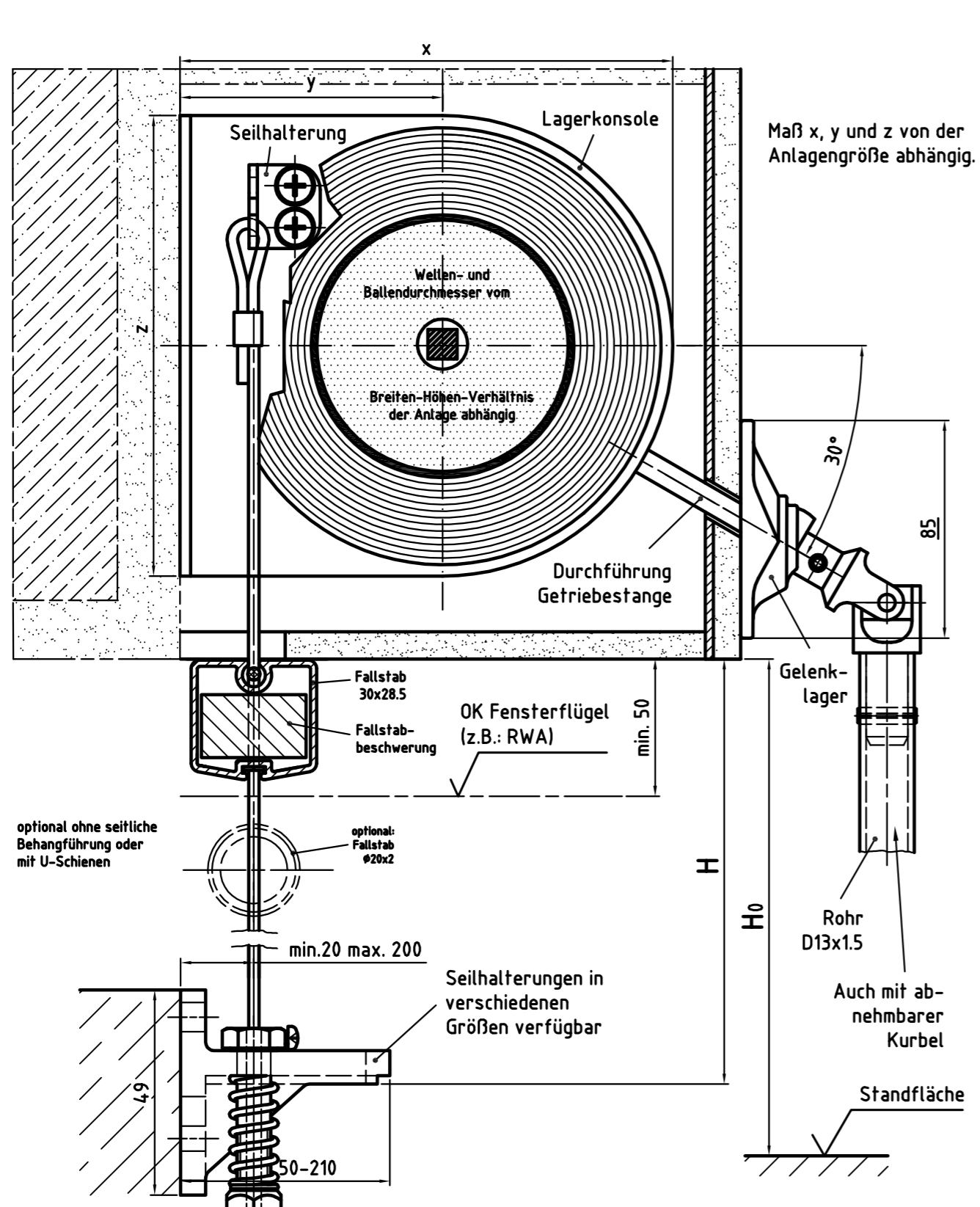
Zeichnung L-GO – Querschnitt Systemskizze | ohne Maßstab | sämtliche Angaben in mm
