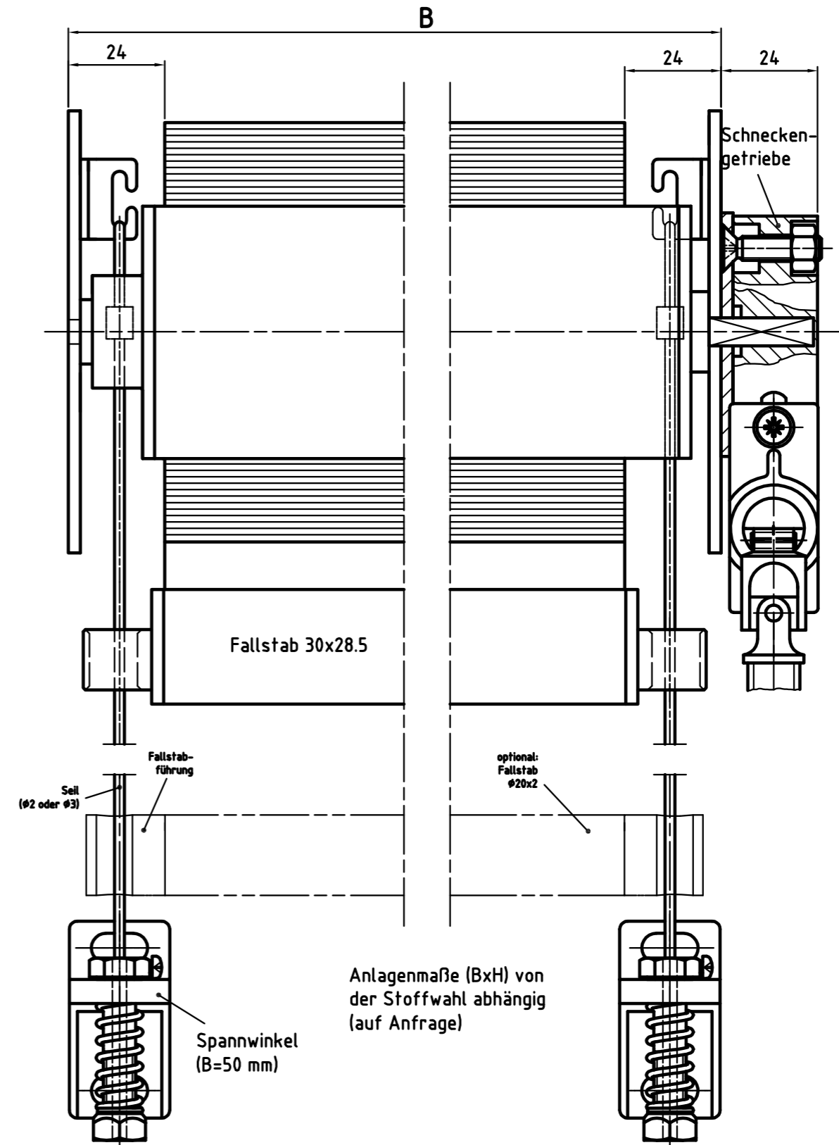
Zeichnung L-GO – Längsschnitt Systemskizze | ohne Maßstab | sämtliche Angaben in mm
