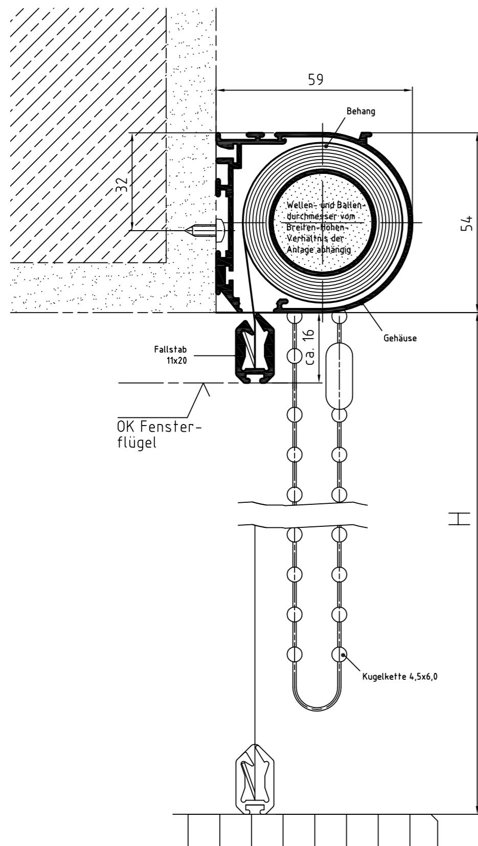
Zeichnung KR 60 – Querschnitt Systemskizze | ohne Maßstab | sämtliche Angaben in mm
