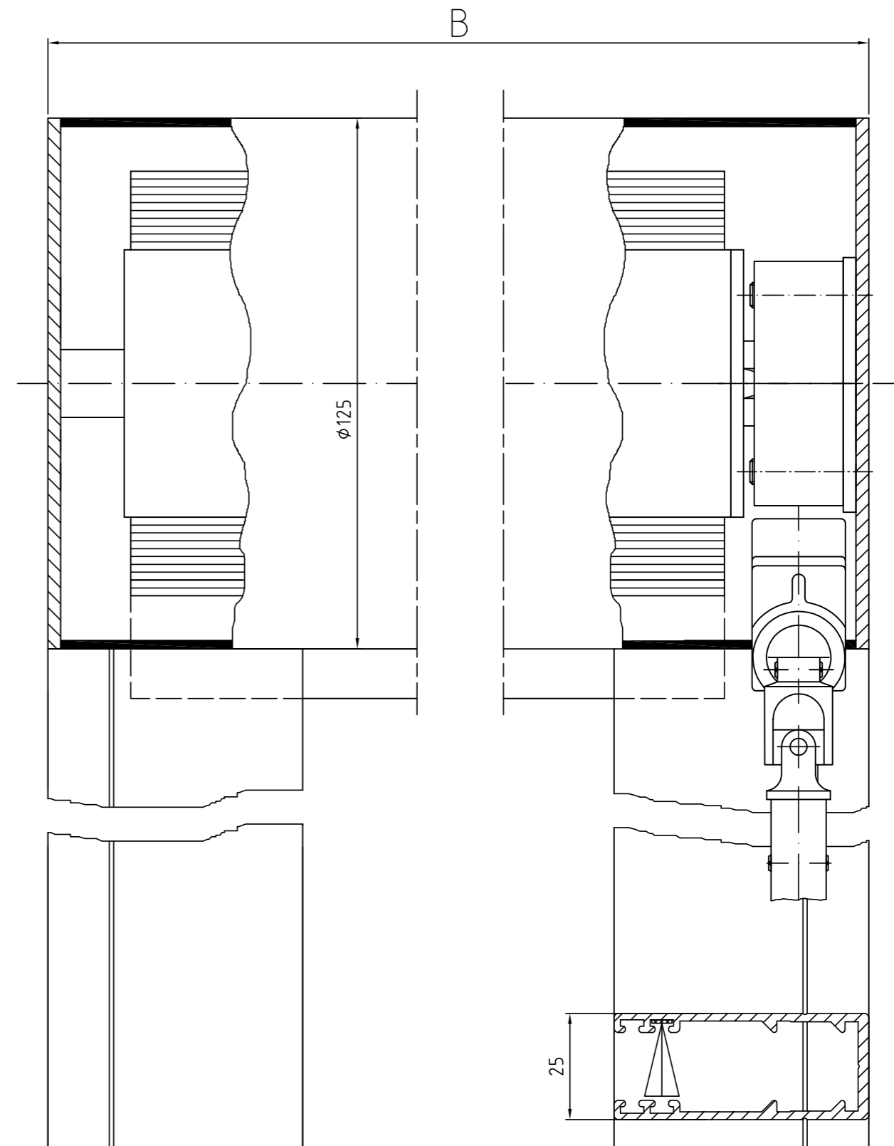
Zeichnung GR 125 – Längsschnitt Systemskizze | ohne Maßstab | sämtliche Angaben in mm
