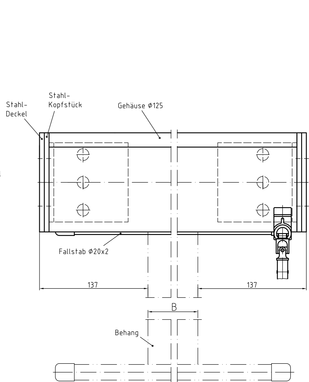
Zeichnung BW-GR 125 – Längsschnitt Systemskizze | ohne Maßstab | sämtliche Angaben in mm
