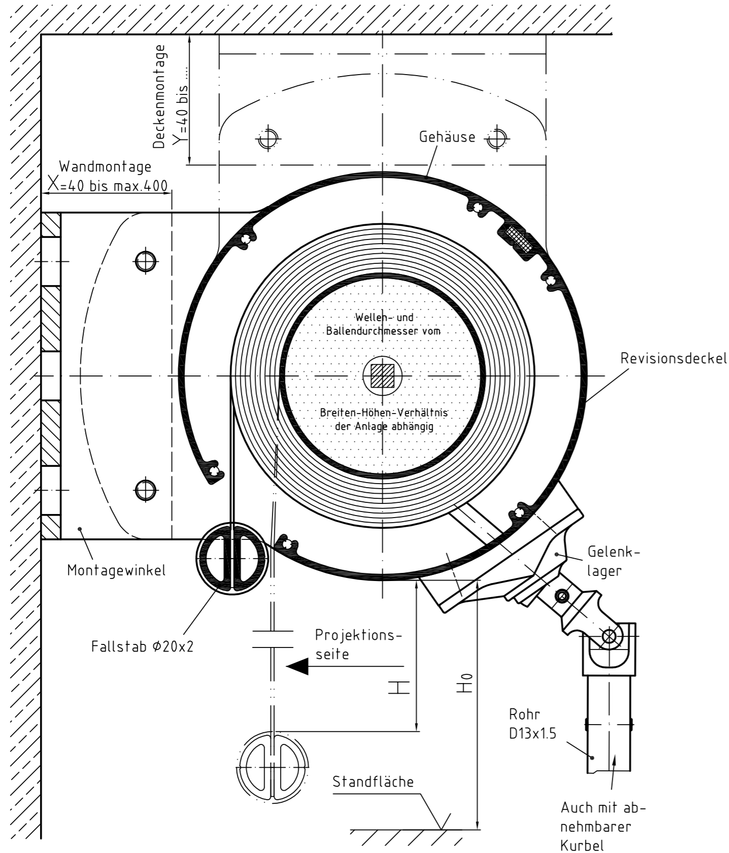
Zeichnung BW-GR 125 – Querschnitt Systemskizze | ohne Maßstab | sämtliche Angaben in mm
